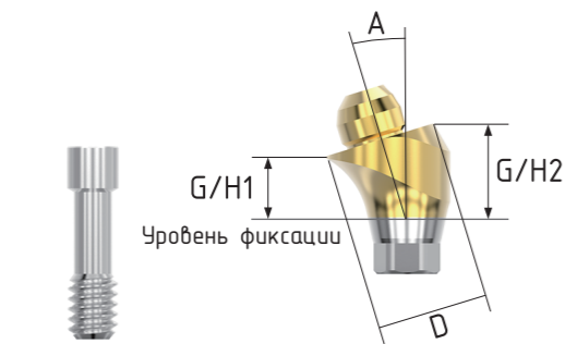
Винт углового абатмента
